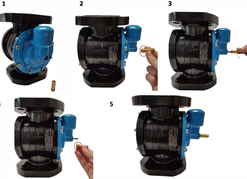
Esempio illustrativo di riarmo e attivazione del dispositivo: Illustrative example of resetting and commissioning of the device:
