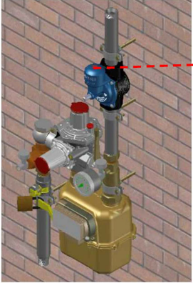
Esempio d'installazione verticale: Vertical installation example:
