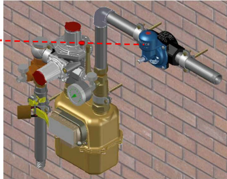
Esempio d'installazione orizzontale: Horizontal installation example:
