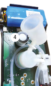
Nouvelle cellule connectée à la carte électronique
