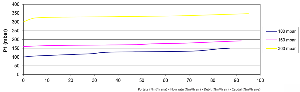
Range 100÷300 mbar
