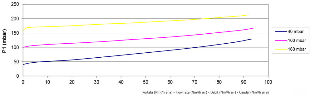
Range 40÷160 mbar
