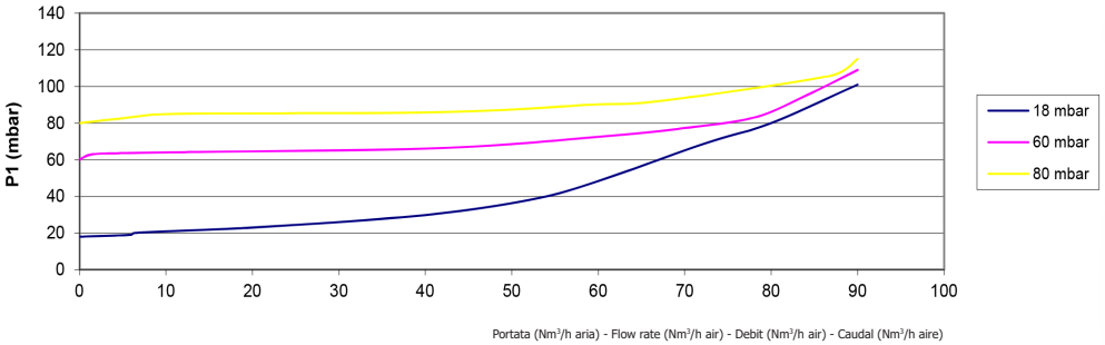
Range 18÷80 mbar
