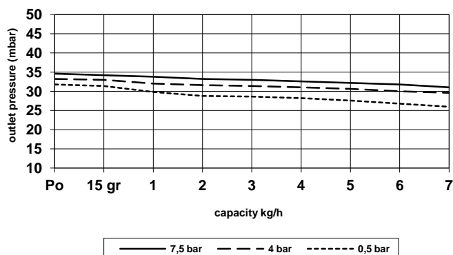
Reg. LP 7 kg/h mod. LPZ 7
