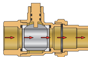
ATTUATORE APERTO
