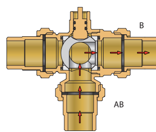
ATTUATORE APERTO
