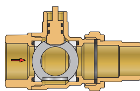
ATTUATORE CHIUSO
